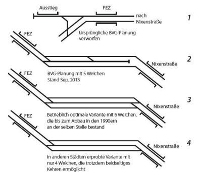
Kehranlage an der Haltestelle FEZ: Die Planungen der BVG (Abb. 1 und 2) und IGEB-Vorschläge dazu (Abb. 3 und 4). Die IGEB-Vorschläge bieten den Vorteil des beidseitigen Wendens und des Abstellens von Arbeits- und Sonderzügen ohne Rangiermanöver - in Abb. 4 sogar mit weniger Weichen als bei der BVG-Planung. (Idee: IGEB, Artur Frenzel, Zeichnung: Stefan Retzlaff)
