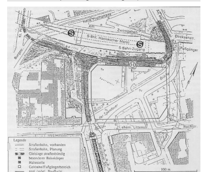
Lageplan-Ausschnitt Spandauer Straße - Stadtbahnviadukt. Maximalen Aufwand plant Senator Haase am S-Bf Hackescher Markt. Heute unterquert die Tram die Stadtbahn westlich des S-Bahnhofs, zukünftig soll sie östlich des S-Bahnhofs fahren, was eine Aufweitung der Stadtbahnbögen erfordert. Und Voraussetzung für die neue Haltestelle wäre ein neuer S-Bahn-Zugang. Den in der Karte eingetragen gibt es nämlich noch gar nicht. (SenVuB: Sachstandsbericht Straßenbahnplanungen, Anlage 1)
