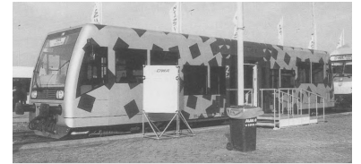
Neuer DWA-Schienenbus auf der InnoTrans, preiswert und mit niedrigem Einsteig, aber mit nur einer Tür und - wie die anderen neuen Nahverkehrstriebwagen auch - ohne WC. (Foto: Thomas Billik (10/96))
